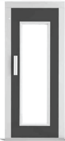
DL4
